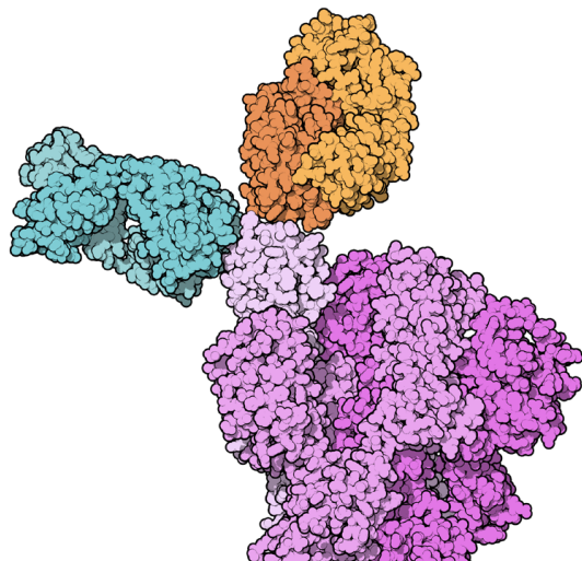
obrázek 2: Modře, oranžově a světle fialově – protilátka, fialově – Spišské protein (jeden z proteinů viru), na který se protilátka váže.
