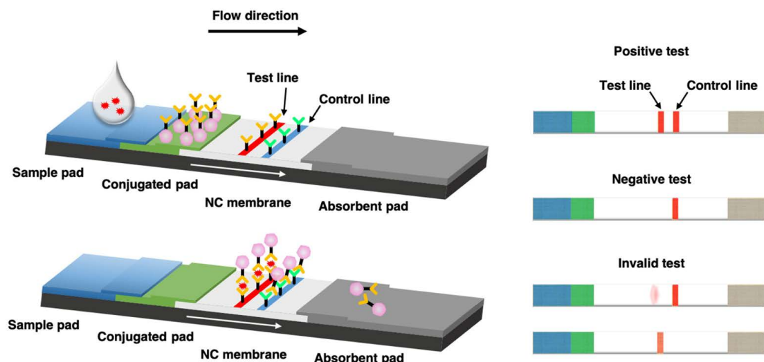
obrázek 1: Princip fungování antigenního testu. Růžově – částice zlata, červeně – částice viru, žlutě – protilátky proti viru, zeleně – protilátky proti protilátkám proti viru.
